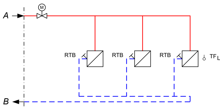
Abbildung 8— Hauszentrale-Raumluftheizung Prinzipschaltbilder für den indirekten Anschluss
