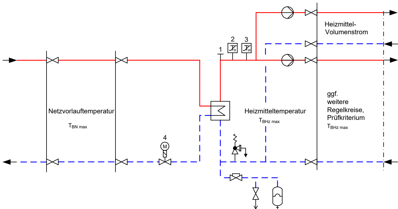
Abbildung zur Tabelle 27 — Erforderliche sicherheitstechnische Ausrüstung
