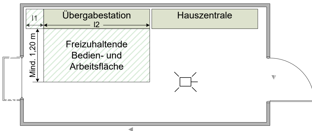
Abbildung 3 — Hausanschlussraum
