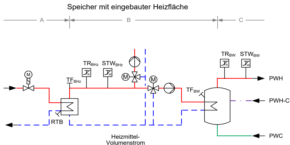
Abbildung 9 — Hauszentrale-Trinkwassererwärmung Prinzipschaltbild für den indirekten Anschluss
