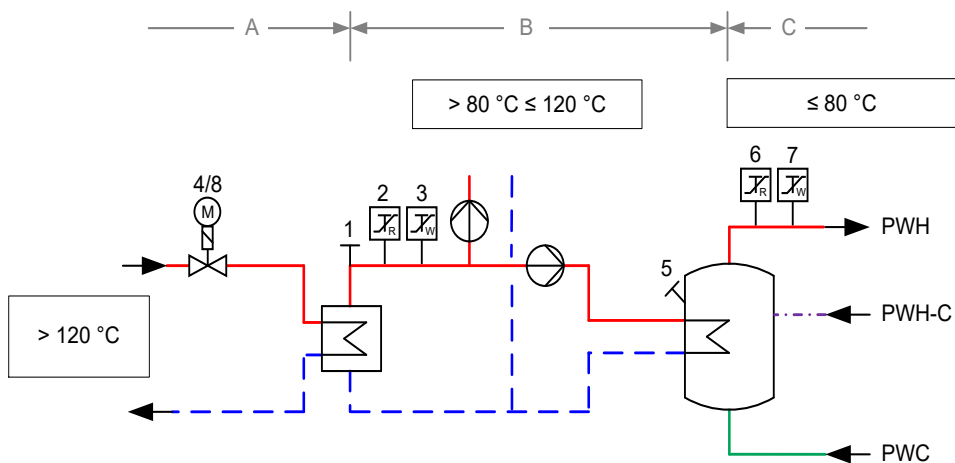
Abbildung zur Tabelle 40 — Erforderliche sicherheitstechnische Ausrüstung nach Zeile 2/3
