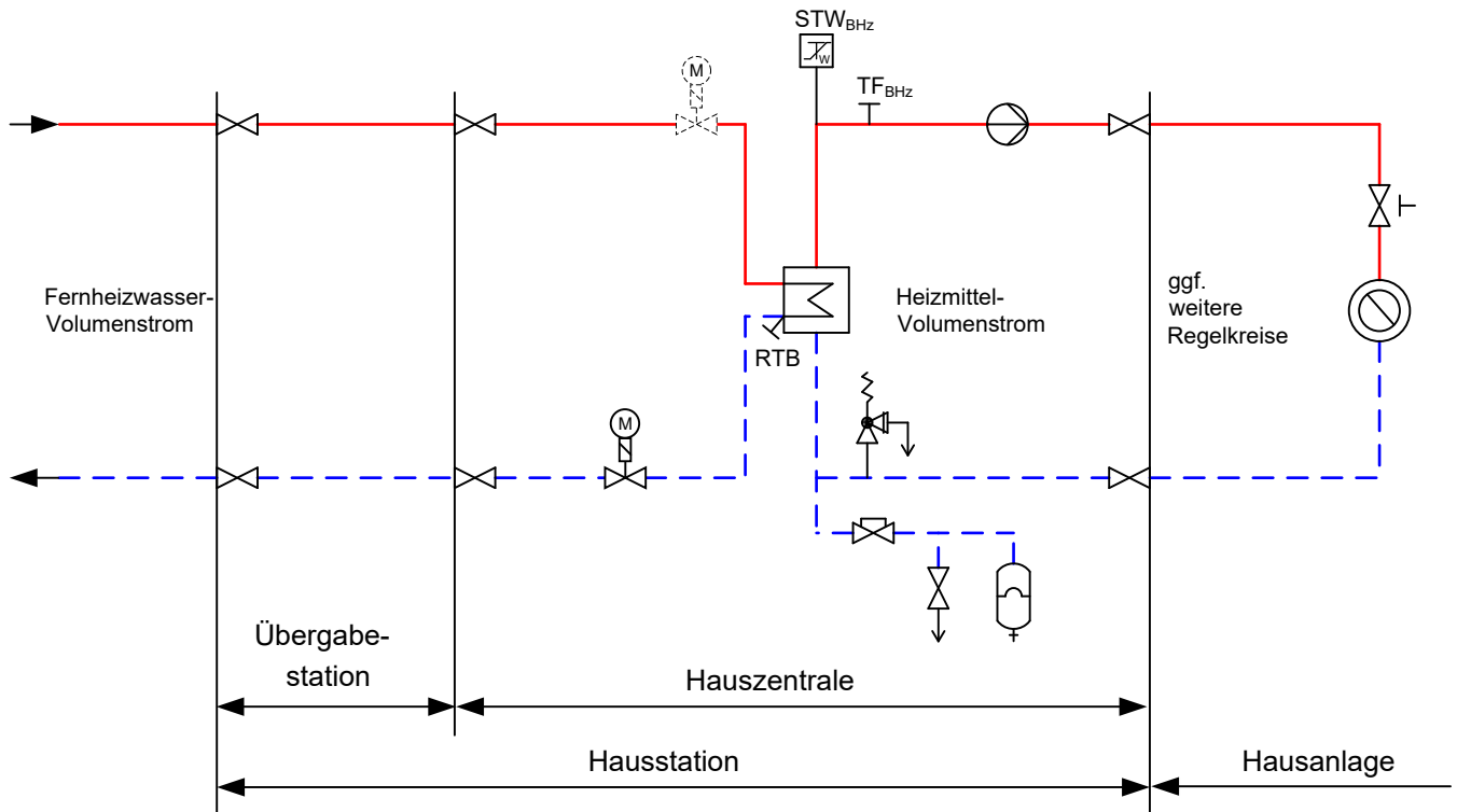
Abbildung 7 Anschluss
