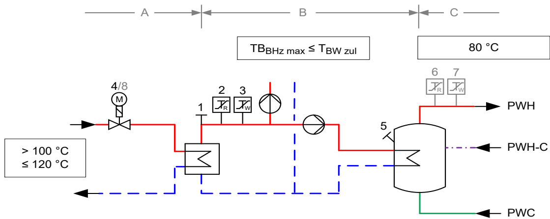
Abbildung zur Tabelle 39 — Erforderliche sicherheitstechnische Ausrüstung nach Zeile 1; grau dargestellte Komponenten nicht erforderlich
