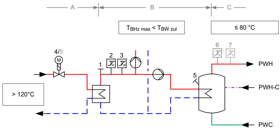
Abbildung zur Tabelle 40 — Erforderliche sicherheitstechnische Ausrüstung nach Zeile 1; grau dargestellte Komponenten nicht erforderlich
