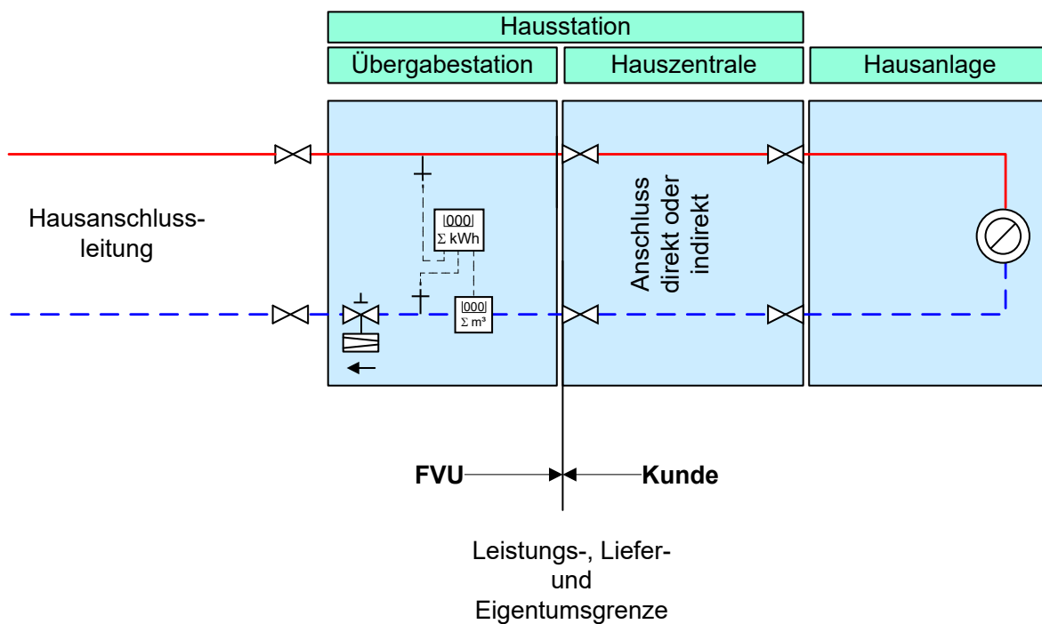
Abbildung 6 — Leistungs-, Liefer- und Eigentumsgrenze
