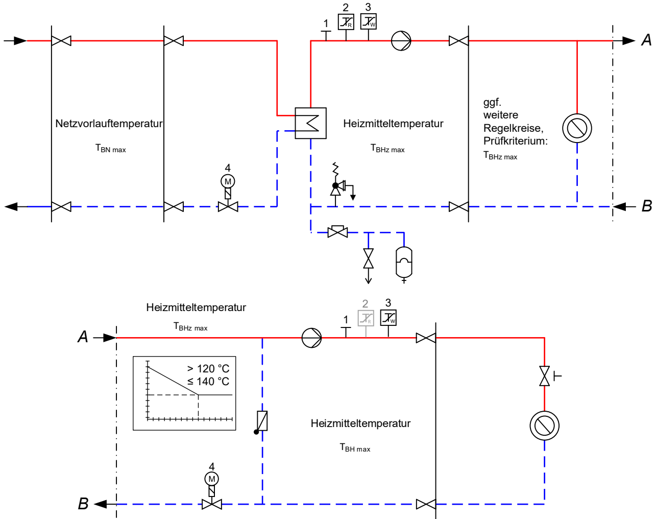
Abbildung zur Tabelle 15 — Erforderliche sicherheitstechnische Ausrüstung nach Zeile 1; grau dargestellte Komponenten nicht erforderlich
