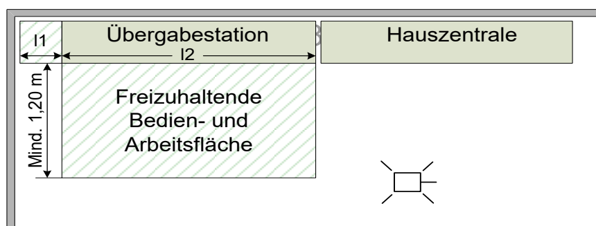
Abbildung 4 – Hausanschlusswand
