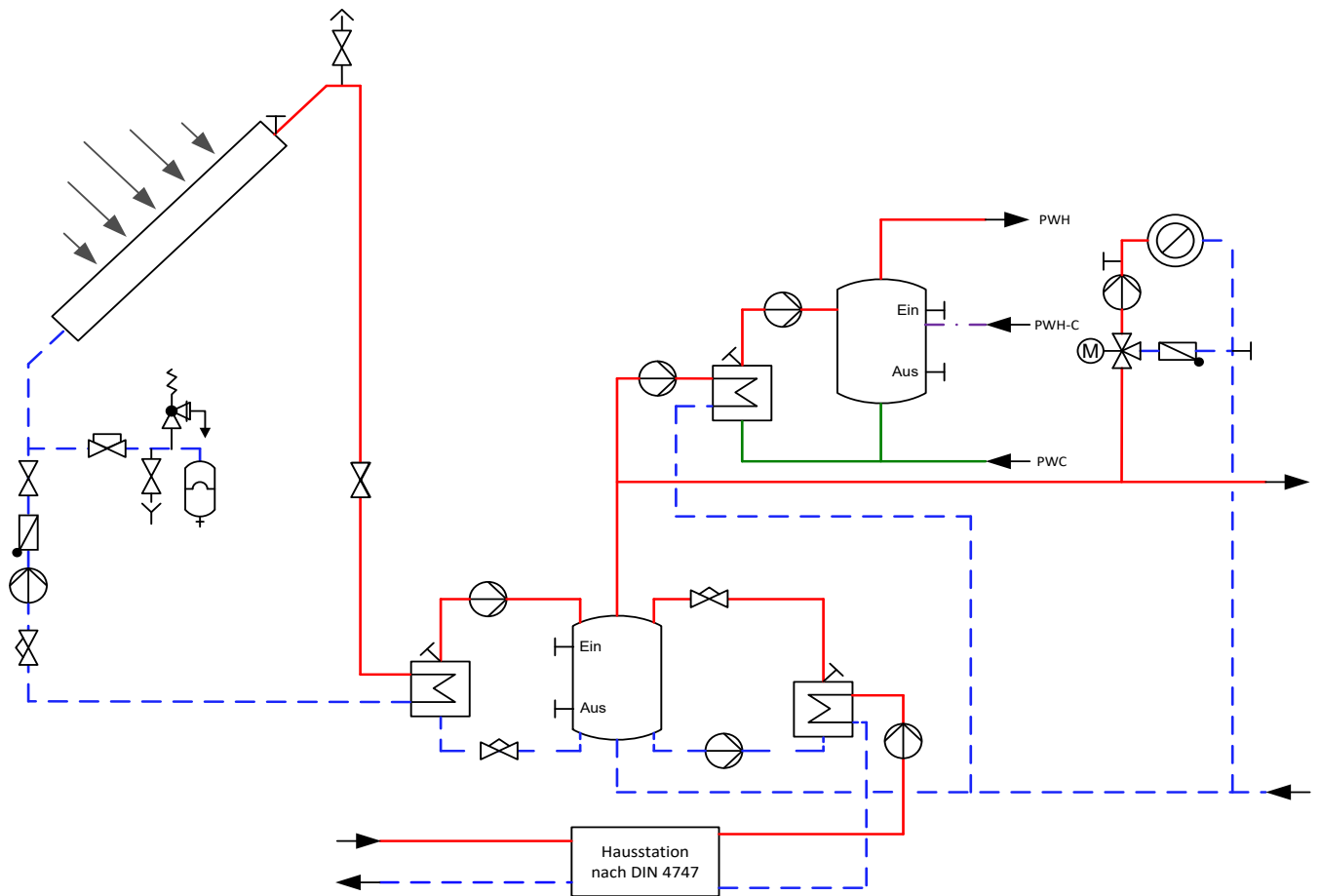
Abbildung 13 — Solar unterstütztes Heizsystem, Pufferspeicher mit außen liegenden Wärmeübertragern für die Solaranlage und die Nachheizung mit Fernwärme
