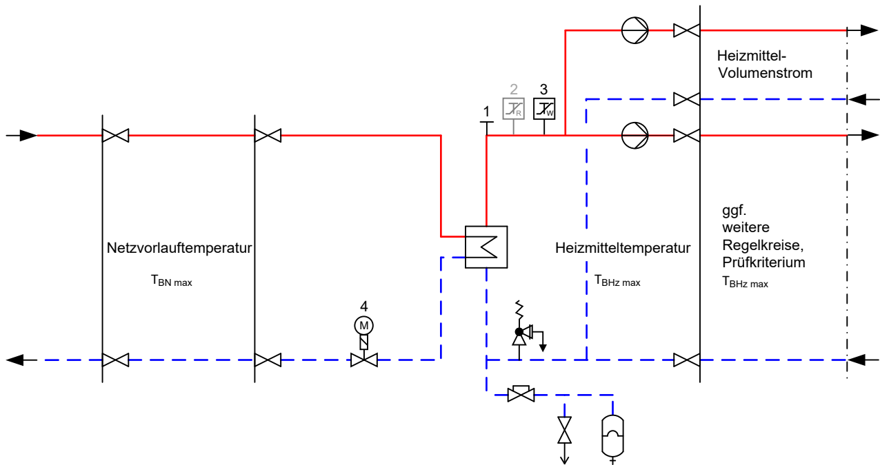
Abbildung zur Tabelle 23 — Erforderliche sicherheitstechnische Ausrüstung nach Zeile 2; grau dargestellte Komponenten nicht erforderlich
