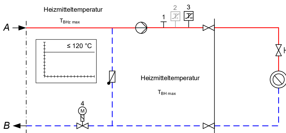
Abbildung zur Tabelle 12 — Erforderliche sicherheitstechnische Ausrüstung nach Zeile 3; grau dargestellte Komponenten nicht erforderlich
