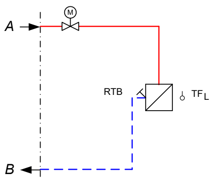
Abbildung 8— Hauszentrale-Raumluftheizung Prinzipschaltbilder für den indirekten Anschluss
