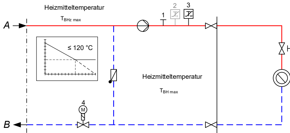
Abbildung zur Tabelle 12 — Erforderliche sicherheitstechnische Ausrüstung nach Zeile 5; 5; grau dargestellte Komponenten nicht erforderlich
