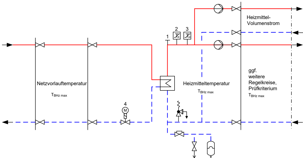
Abbildung zur Tabelle 24 — Erforderliche sicherheitstechnische Ausrüstung
