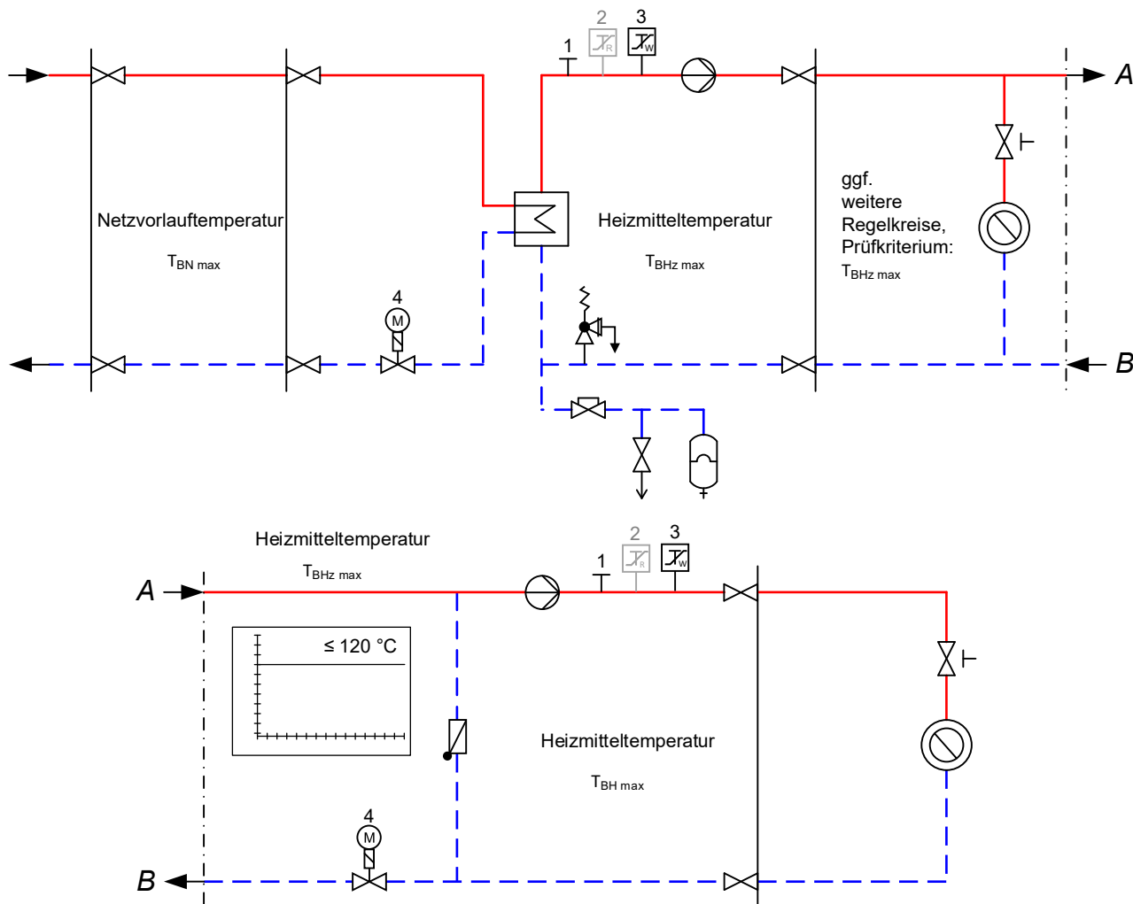
Abbildung zur Tabelle 14 — Erforderliche sicherheitstechnische Ausrüstung nach Zeile 2; grau dargestellte Komponenten nicht erforderlich
