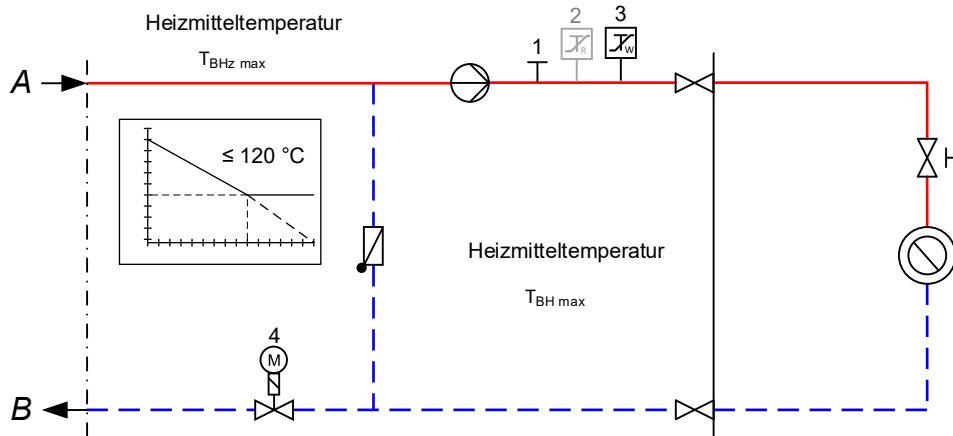
Abbildung zur Tabelle 15 — Erforderliche sicherheitstechnische Ausrüstung nach Zeile 5; grau dargestellte Komponenten nicht erforderlich
