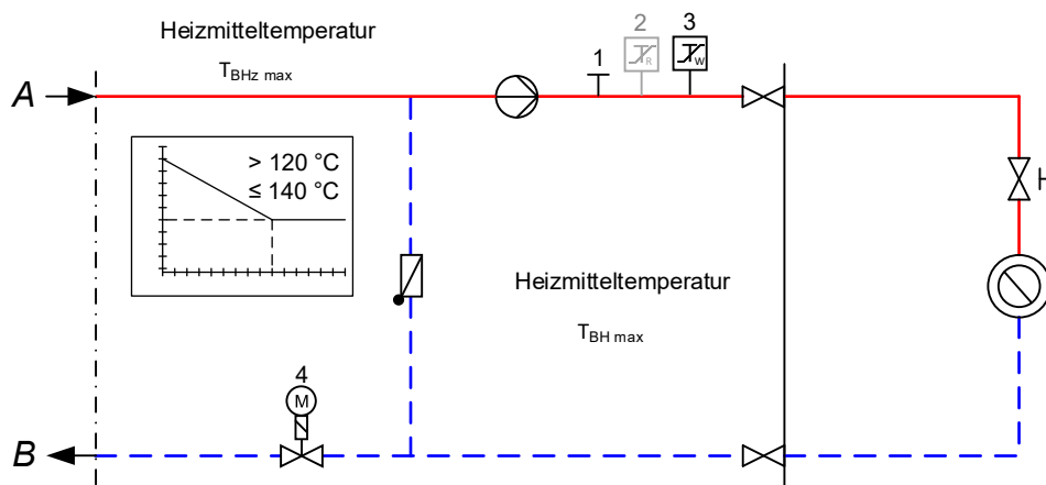
Abbildung zur Tabelle 12 — Erforderliche sicherheitstechnische Ausrüstung nach Zeile 1; grau dargestellte Komponenten nicht erforderlich
