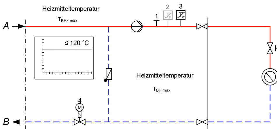
Abbildung zur Tabelle 15 — Erforderliche sicherheitstechnische Ausrüstung nach Zeile 3; grau dargestellte Komponenten nicht erforderlich
