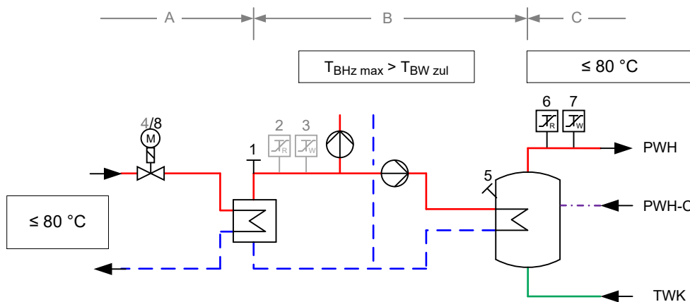
Abbildung zur Tabelle 37 — Erforderliche sicherheitstechnische Ausrüstung nach Zeile 2; grau dargestellte Komponenten nicht erforderlich
