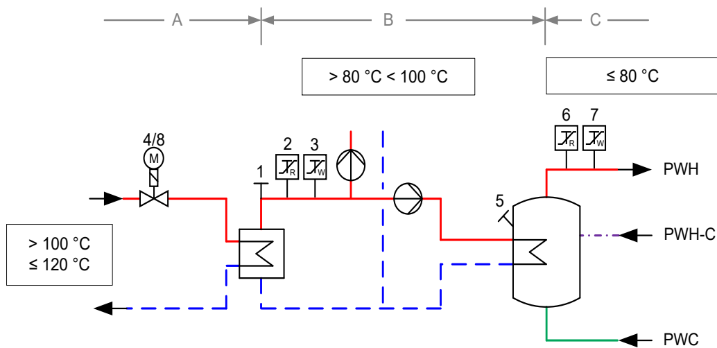
Abbildung zur Tabelle 39 — Erforderliche sicherheitstechnische Ausrüstung nach Zeile 2; grau dargestellte Komponenten nicht erforderlich
